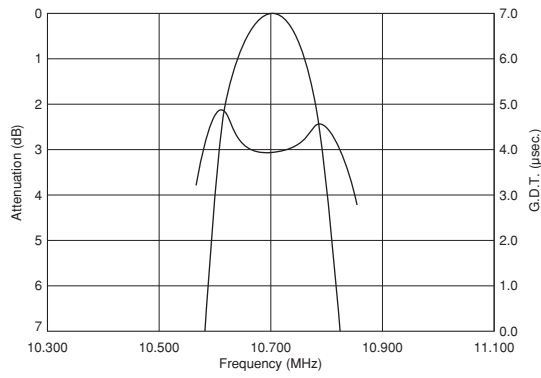
SFECF10M7HA00-R0/SFECF10M7HF00-R0
