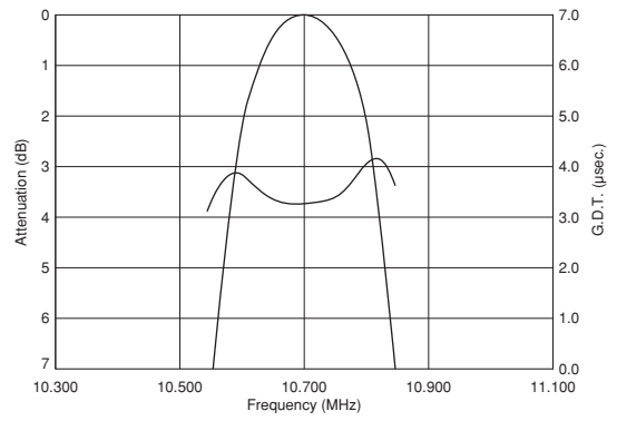
SFECF10M7GA00-R0/SFECF10M7GF00-R0
