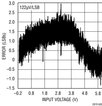
ADC INL
